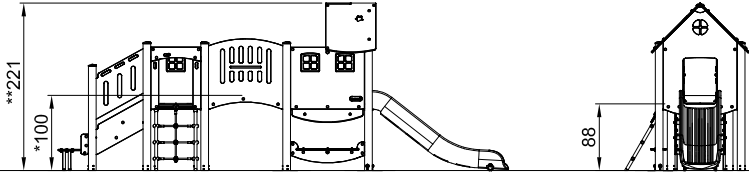
PCM200204 1:100
