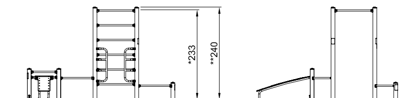
FSW10200 1:100
