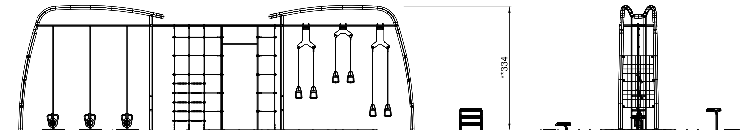
FSP30100 1:100
